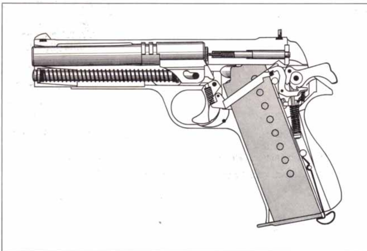
Vue en coupe d'un P 210-1 ou P 210-2
